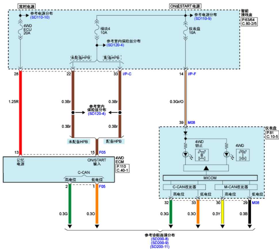
分动器控制系统(TCCS)(1)
